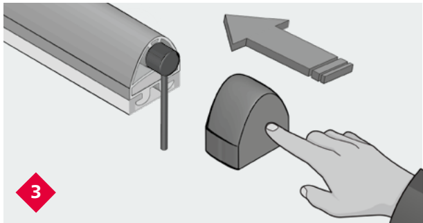
Gummiprofil einziehen / Endkappen stecken
