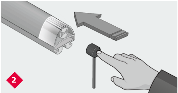
Sensor / Widerstand stecken
